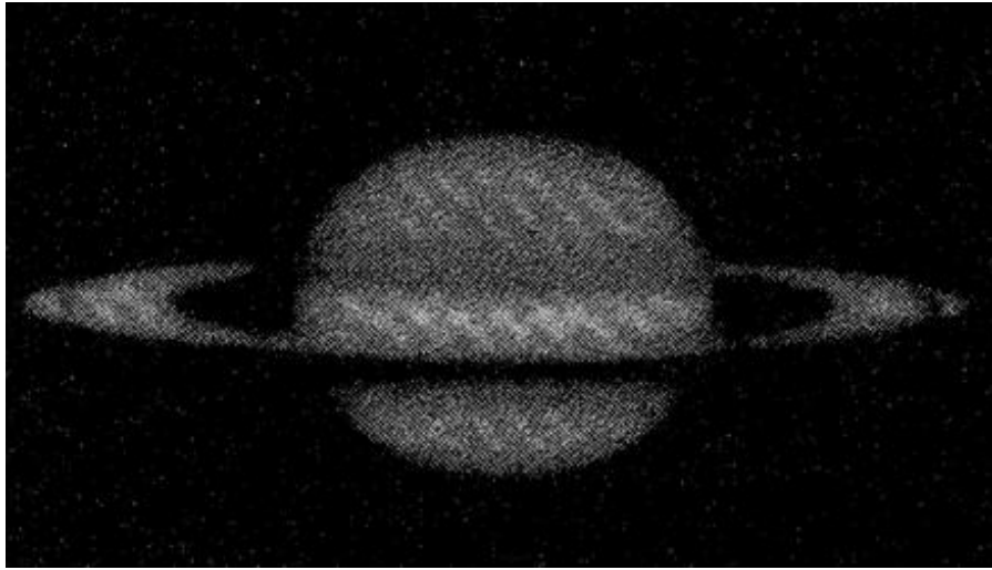
FIG. 4. SATURN.
